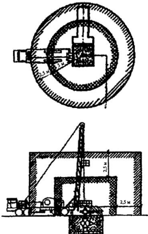
Рис.9. Агрегат для ремонта скважин
