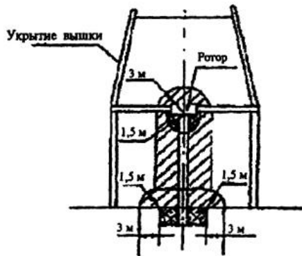
Буровая установка с открытым подроторным пространством
