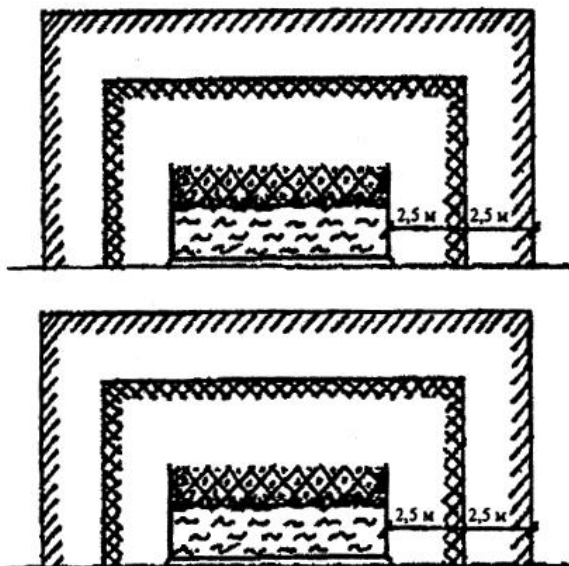
Рис.4. Открытые пространства вокруг открытых емкостей, аппаратов, устройств
