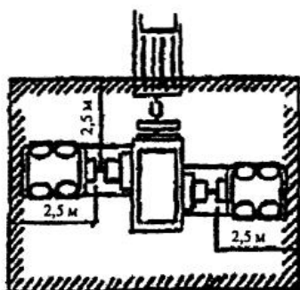
Газовый компрессор
