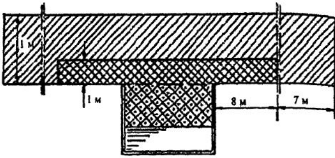
Рис.7. Открытые пространства вокруг открытого сепаратора
