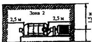
Насос для перекачки нефти
