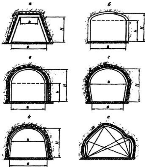
Рис.2. Поперечные сечения горных выработок:
